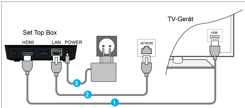
Abbildung 2: Kabelverbindungen
